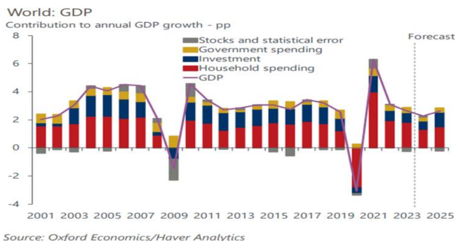
Рисунок 1 – Мировой ВВП [2]
