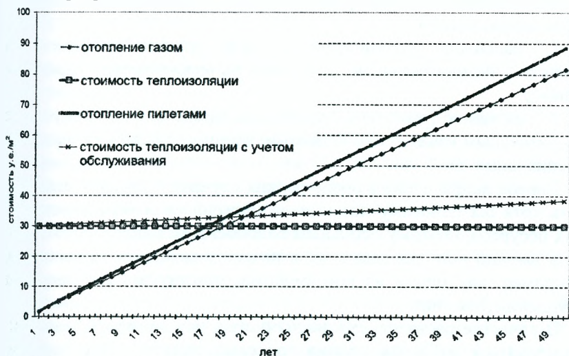
Рис. 1. Соотношение стоимости создания и обслуживания полимерной или ячеистобетонной теплоизоляции со стоимостью сэкономленных энергоресурсов при отоплении древесными пилетами или газом
