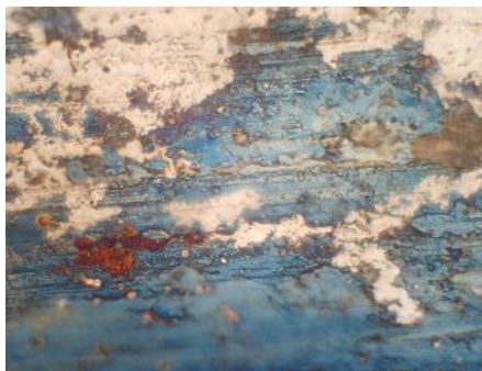
Рис. 7. Оксидная пленка на поверхности покрытия после МЭШ
