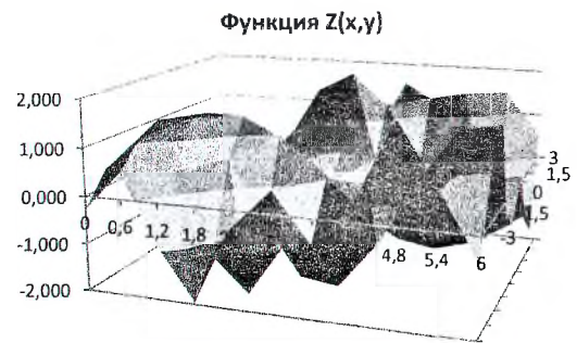
Рисунок 3 – Поверхностная диаграмма
