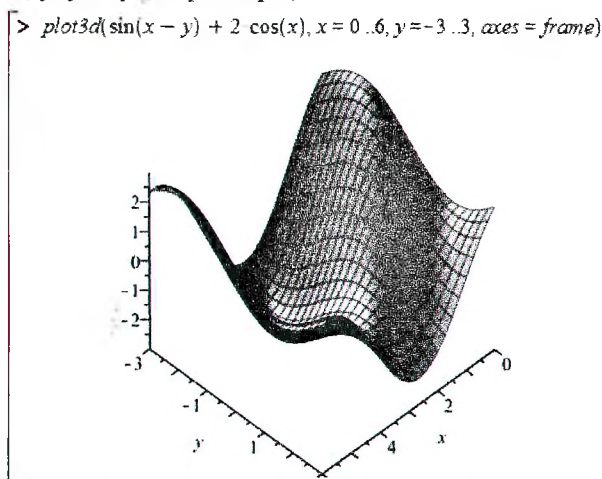
Рисунок 25 – Пространственный график
