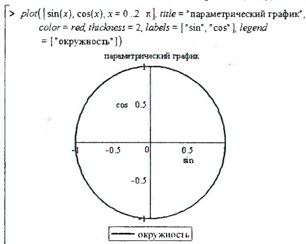
Рисунок 24 – Параметрический график
