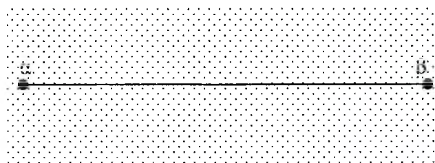
метод золотого сечения
