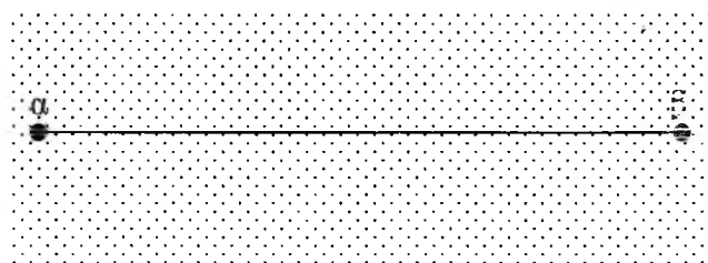
метод дихотомии
