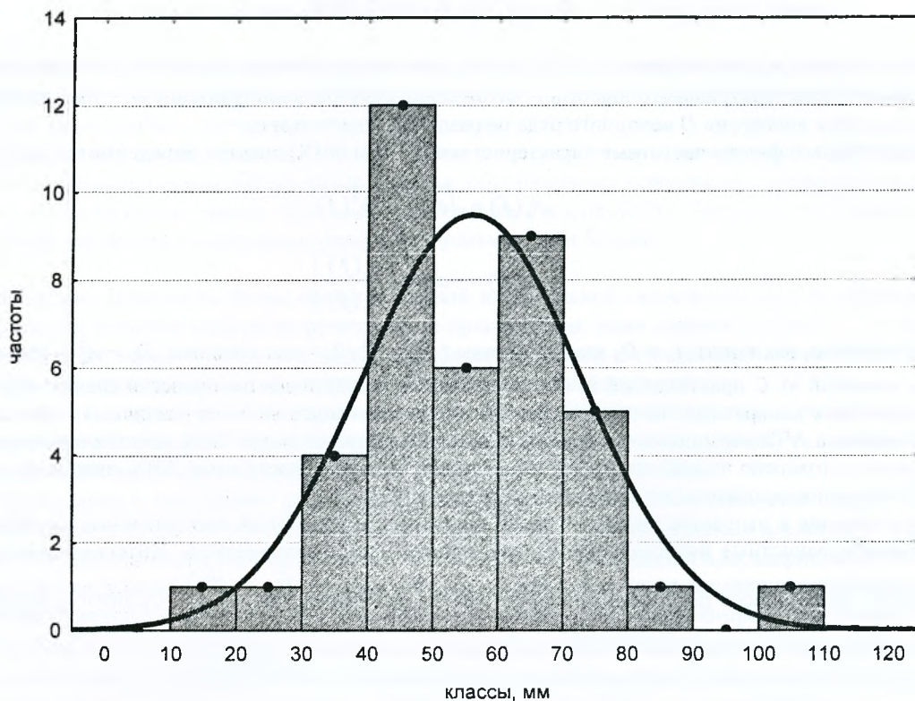
Рис. 1. Гистограмма распределения средних за вегетационный период продуктивных влагозапасов (ст. Василевичи)
