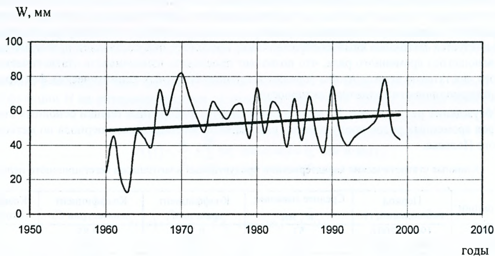
Рис. 2. Гидрограф продуктивных влагозапасов минеральных почв ст. Василевичи
