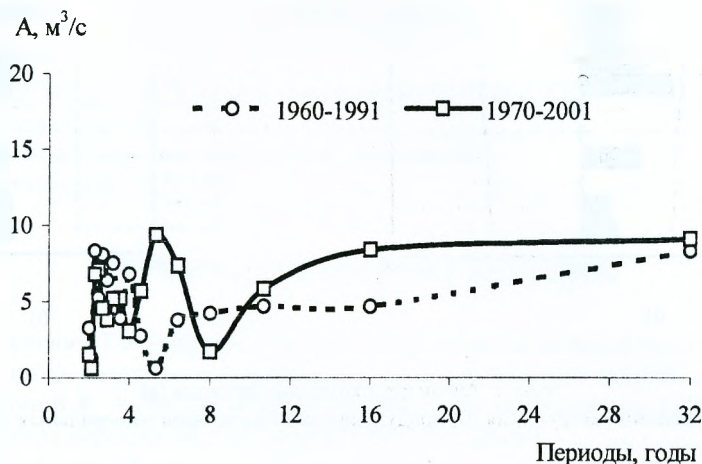
Рис. 3. Периодограммы продуктивных влагозапасов за 1960 – 1991 и 1970 – 2001 годы
