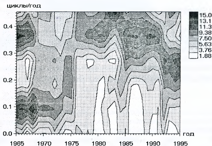
Рис. 6. СВАН-диаграмма продуктивных влагозапасов ст. Василевичи (длина скользящего окна 11 лет)
