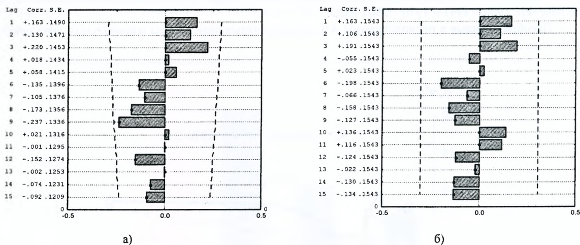
Рис. 5. Автокорреляционная функция (а) и частная автокорреляционная функция (б) продуктивных влагозапасов минеральных почв ст. Василевичи
