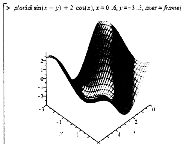
Рисунок 25 – Пространственный график
