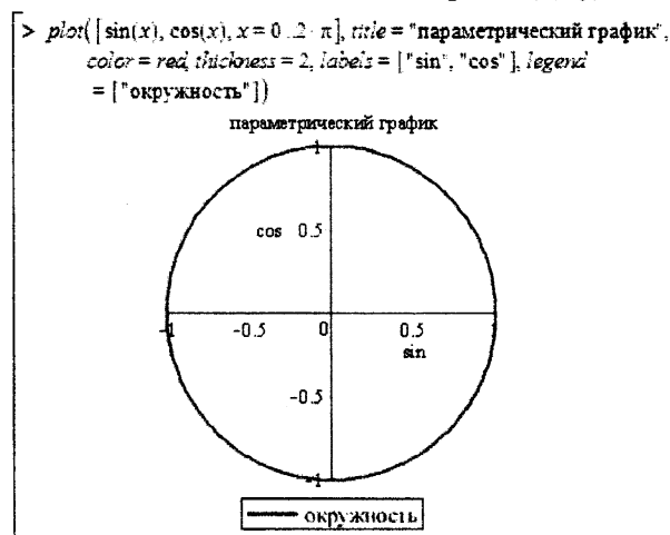
Рисунок 24 – Параметрический график
