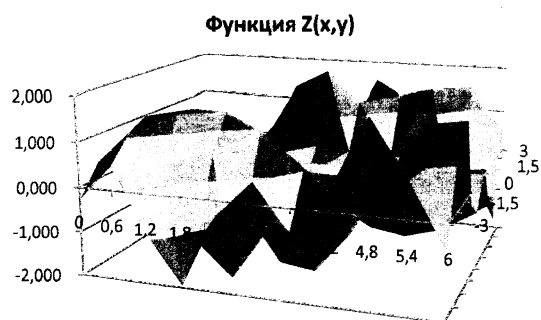
Рисунок 3 – Поверхностная диаграмма
