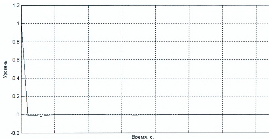
Рис. 2. Обобщенная автокорреляционная функция сигналов шумовых диодов
