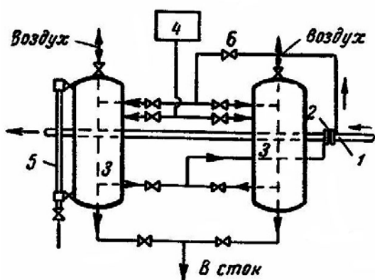
Рисунок 3.2 – Схема установки шайбовых дозаторов
