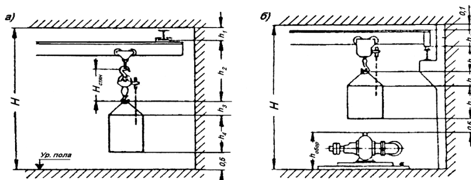
Рисунок 10.1 – Схемы размещения грузоподъемных устройств внутри сооружений
