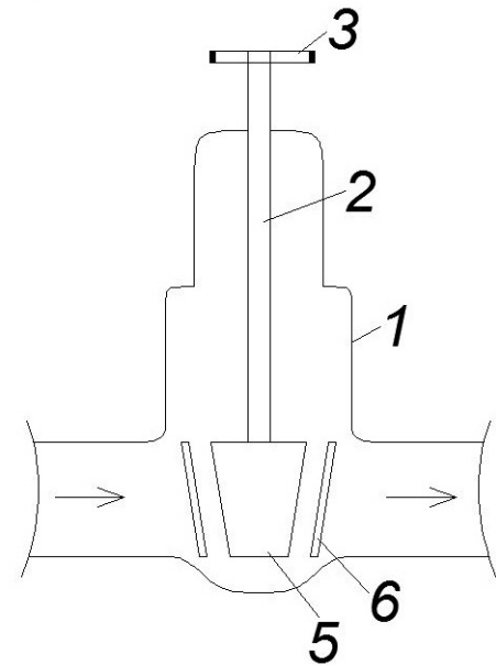
а) Клиновая задвижка
