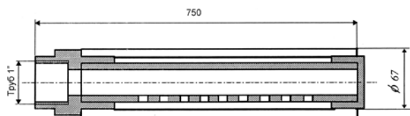
Рисунок 8.4 – Трубчатый аэратор с перфорированной эластичной мембраной
