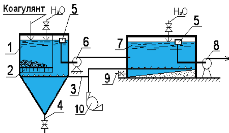
Рисунок 2.1 – Схема приготовления раствора коагулянта с “сухим” хранением реагента
