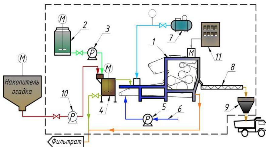
Рисунок 9.4. - Типовая технологическая схема процесса механического обезвоживания осадка [13]
