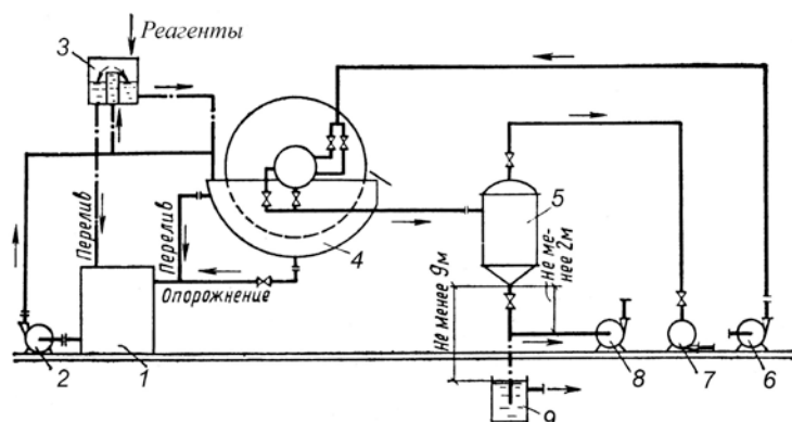
Рисунок 9.5 – Типовая схема установки барабанного вакуум-фильтра
