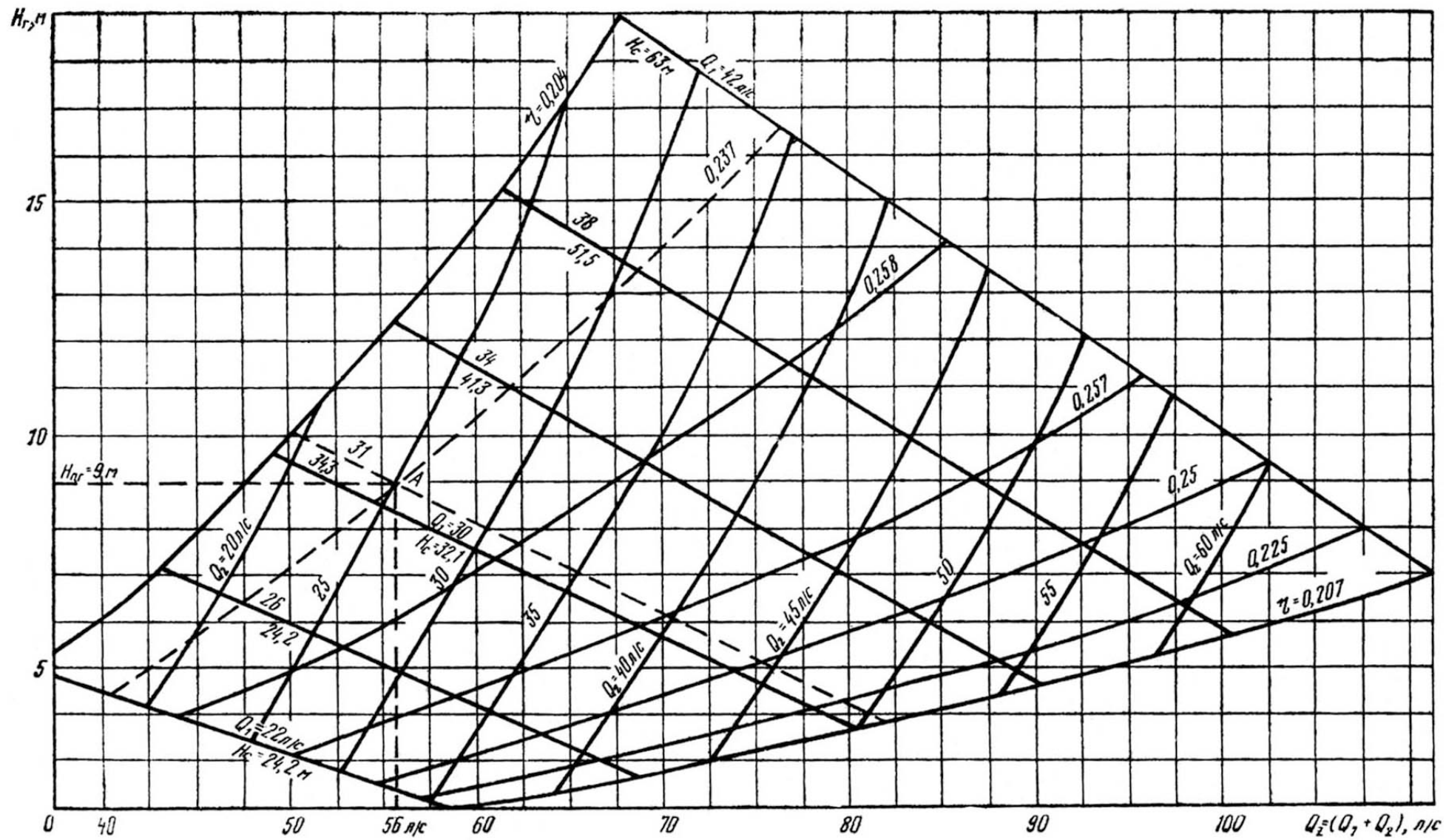
Рисунок 7.3 – Характеристика стационарного гидроэлеватора при d_c = 40 мм и d_z = 80 мм
