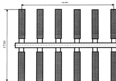
Рисунок 8.5 – Базовый вариант секции аэраторов
