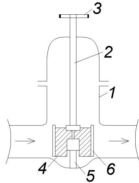
б) Параллельная задвижка
