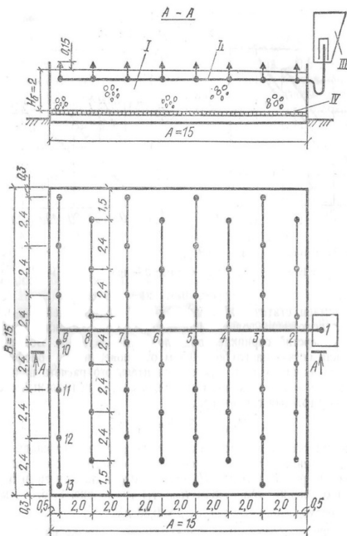
Рисунок 8.1 - Водораспределительная сеть капельного биофильтра:
