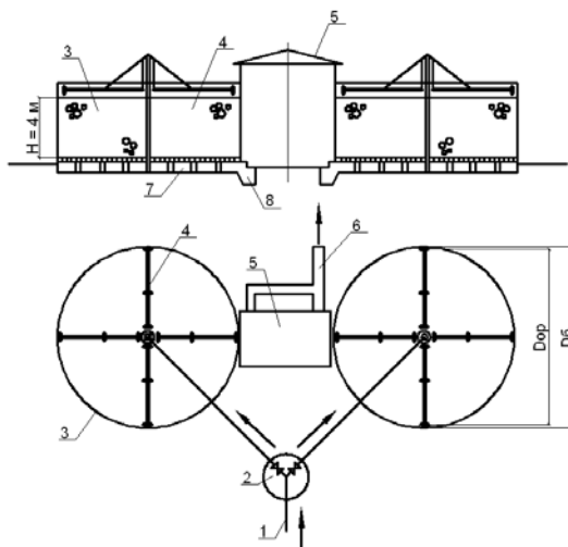
Рисунок 8.3 – Высокнагружаемые биофильтры (аэрофильтры) с реактивными оросителями
