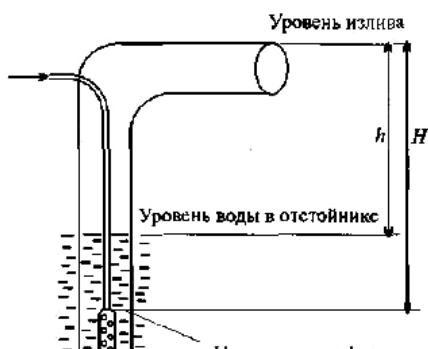
Рисунок 7.4 – Схема эрлифта с расположением форсунки внутри пульпоподъемной трубы
