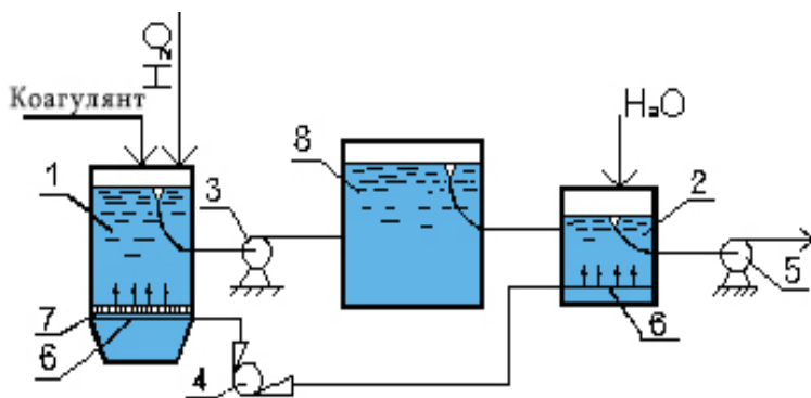
Рисунок 2.2 – Схема приготовления раствора коагулянта с “мокрым” хранением реагента
