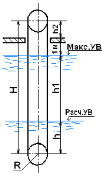
Рисунок 6.1 – Схема для гидравлического расчета вращающейся сетки
