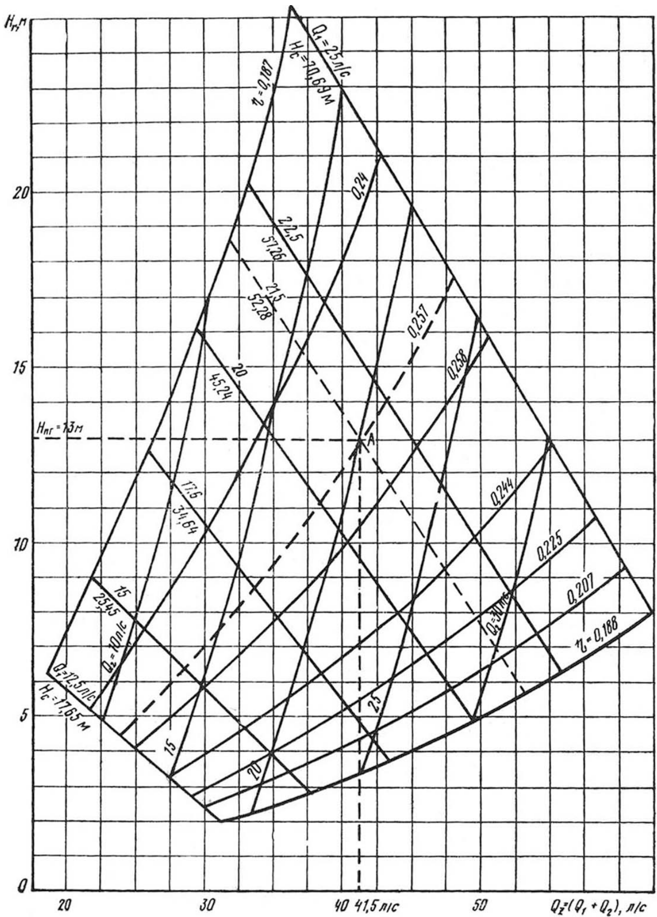
Рисунок 7.2 – Характеристика стационарного гидроэлеватора при d_c = 30 мм и d_2 = 55 мм
