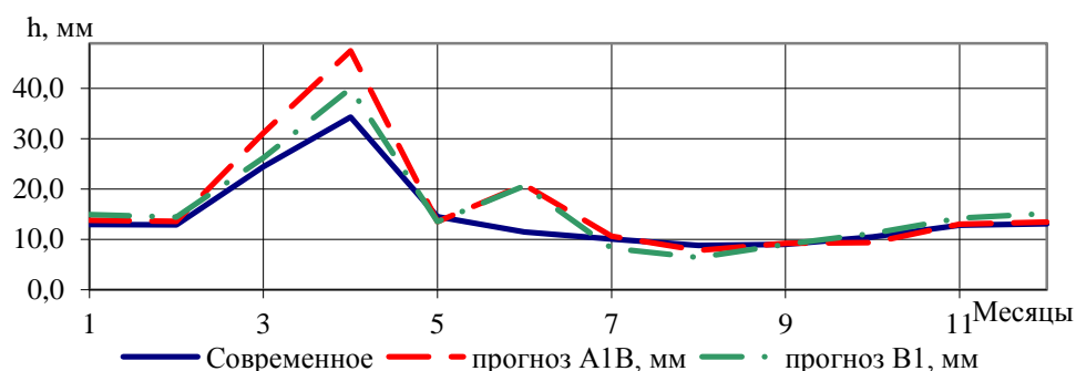
Рисунок 5 – Гидрографы годового стока р. Неман в створе г. Столбцы для различных сценариев климата.
