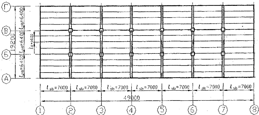
Рисунок 2 а — 1-ый вариант компоновки перекрытия
