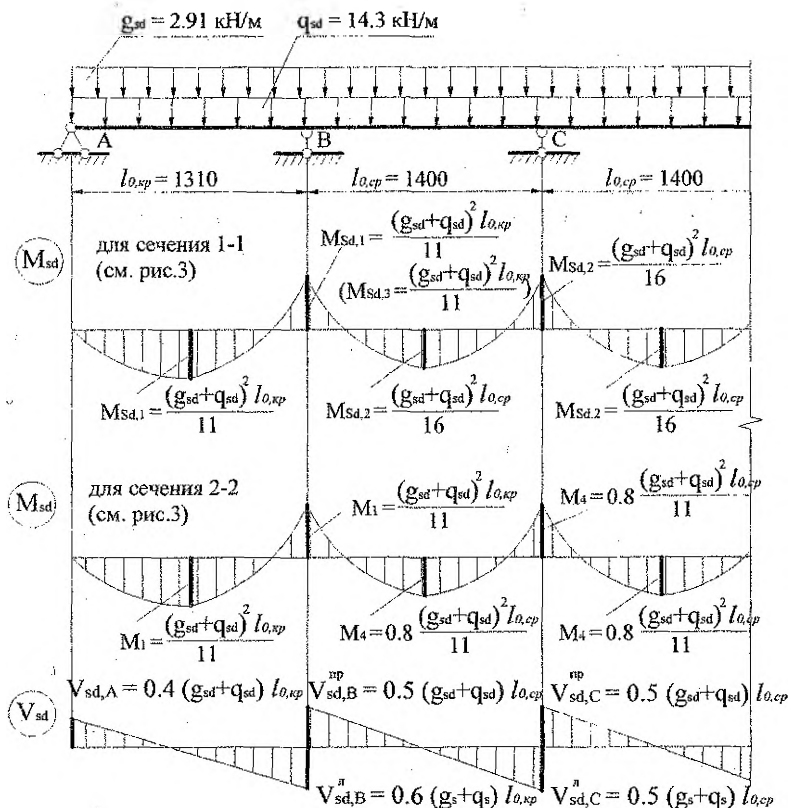
Рисунок 5 — Расчетная схема монолитной плиты с эпюрами усилий
