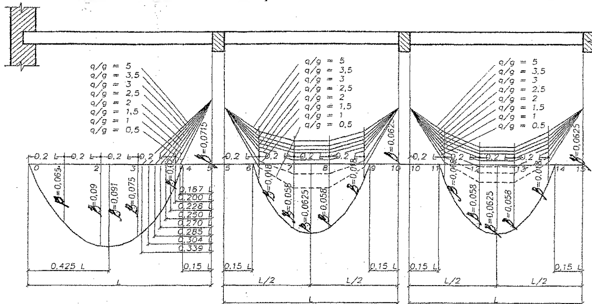
Рисунок 5-1 – Элюры расчетных моментов для равнопролетных неразрезных второстепенных балок
