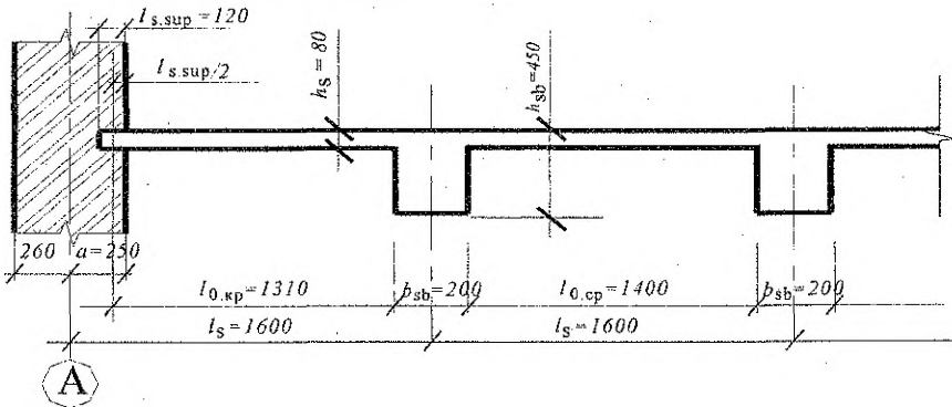
Рисунок 4 — К определению расчетных пролетов монолитной плиты
