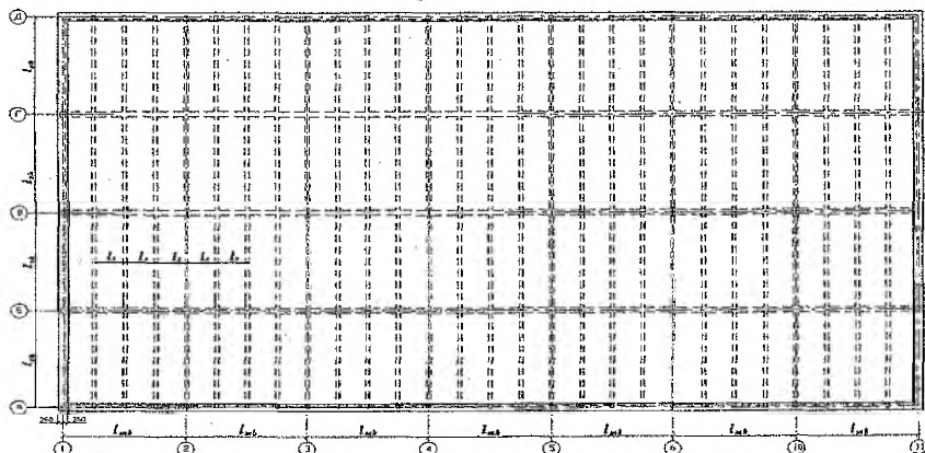
Рисунок 1 — К назначению размеров пролетов и поперечных сечений элементов монолитного перекрытия
