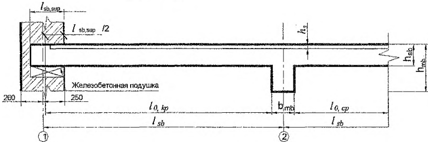
Рисунок 8 – К определению расчетных пролетов второстепенной балки
