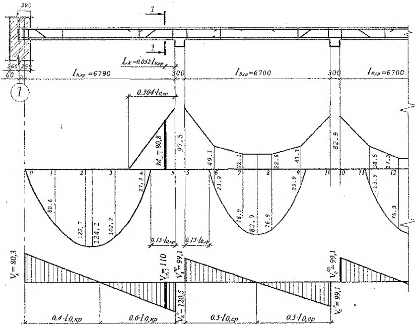
Рисунок 10 – Расположение расчетных сечений для второстепенной балки
