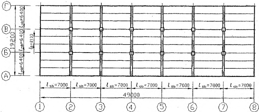
Рисунок 2 в — 3-ий вариант компоновки перекрытия
