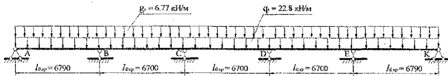
Рисунок 9 – Расчетная схема второстепенной балки
