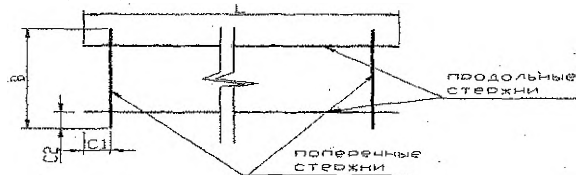
Рисунок 7 – К конструированию сеток
