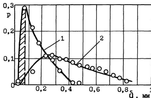
Рис. 3. Частота p распределения биений \delta рабочего торца маховика двигателя ЗМЗ-53 относительно оси коренных шеек коленчатого вала. Сборочная единица собрана из необезличенных (1) и обезличенных (2) деталей
