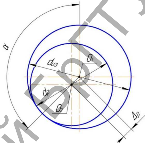
Рис. 2. Схема расположения контура шатунной шейки вала после обработки диаметром d_p в контуре шейки до обработки диаметром d_{из} . Обозначения: O_1 – центр окружности изношенной шейки; O_2 – центр окружностей, совпадающий с осью вращения шпинделя станка; \alpha – угол между линией центров окружностей и осью кривошипа; \Delta_p – геометрическая сумма отклонений расположения и формы обрабатываемой поверхности
