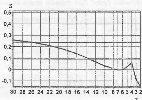
Рисунок 2. – Типовой для второй группы спектр уровня озера Лукомское
