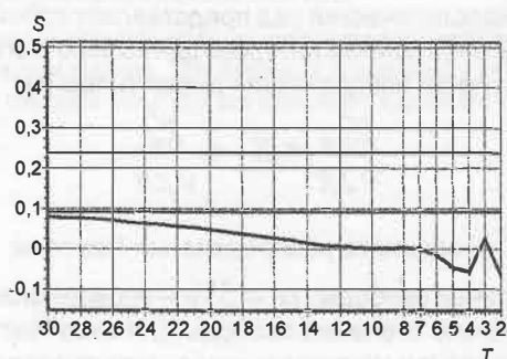
Рисунок 3. – Типовой для третьей группы спектр уровня озера Łebsko
