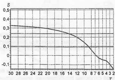
Рисунок 1. – Типовой для первой группы спектр уровня озера Выгоноцанское
