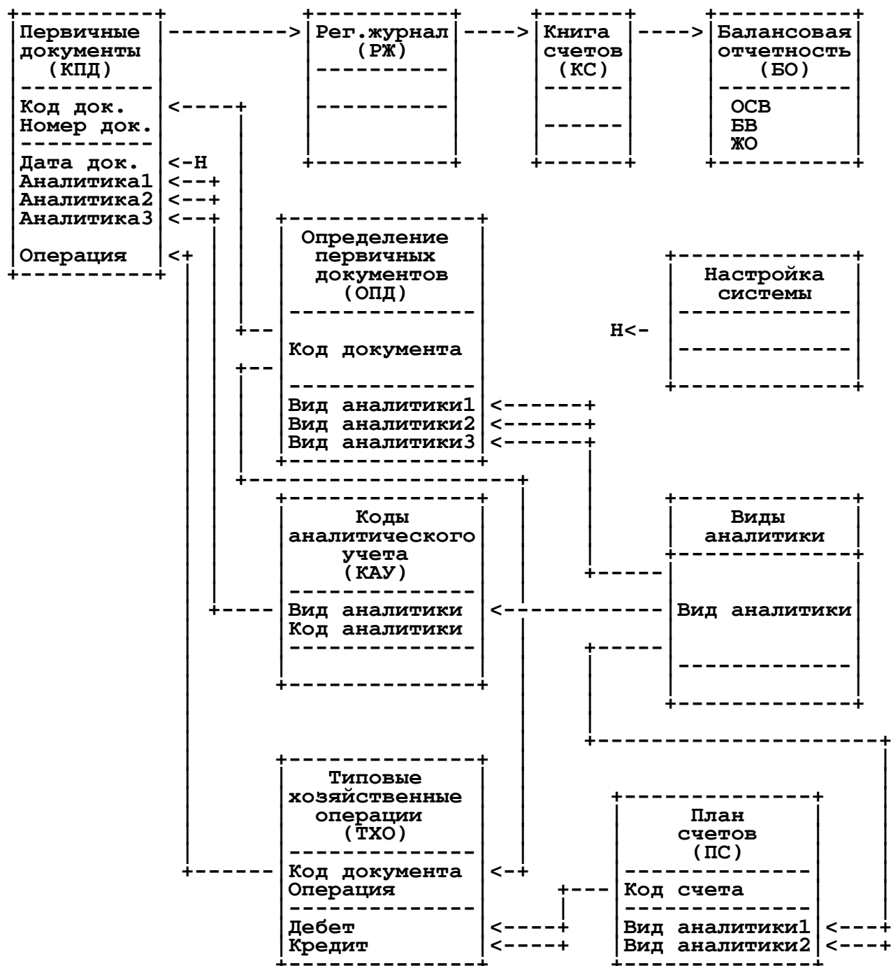
Рис. 3.1. Схема обработки данных АРМ'а «Баланс предприятия»
