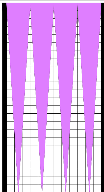
Рис. 2. Обтекание плоской водяной струей сетчатого экрана с размером ячейки 10×10 мм ( q_{уд}=1 л/с на пог.м)
