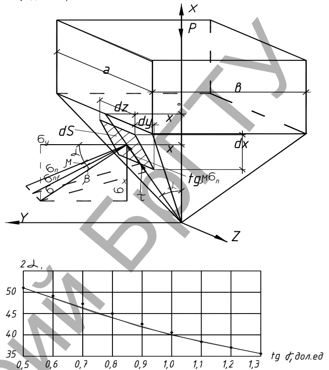
Рис. 1. Расчетная схема раскладки напряжений при минимальном сопротивлении грунта под сваями (а) и график зависимости оптимальных углов заострения сваи 2\alpha в зависимости от tg \gamma (б)
