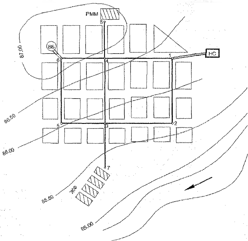
Рис. 2.1 – Трассировка водопроводной сети
