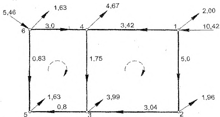
Рис. 3.1 – Предварительное потокораспределение
