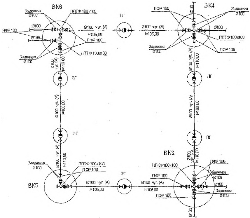
Рис. 8.1 – Детализровка водопроводного кольца № 2
