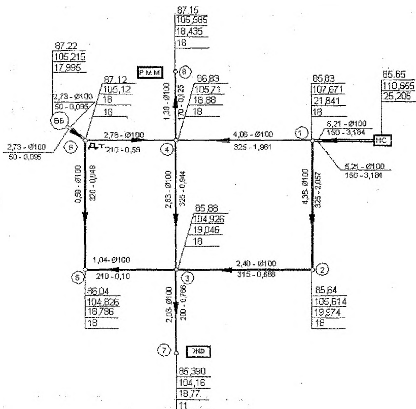
Рис. 3.2 – Расчет пьезометрических отметок и свободных напоров
