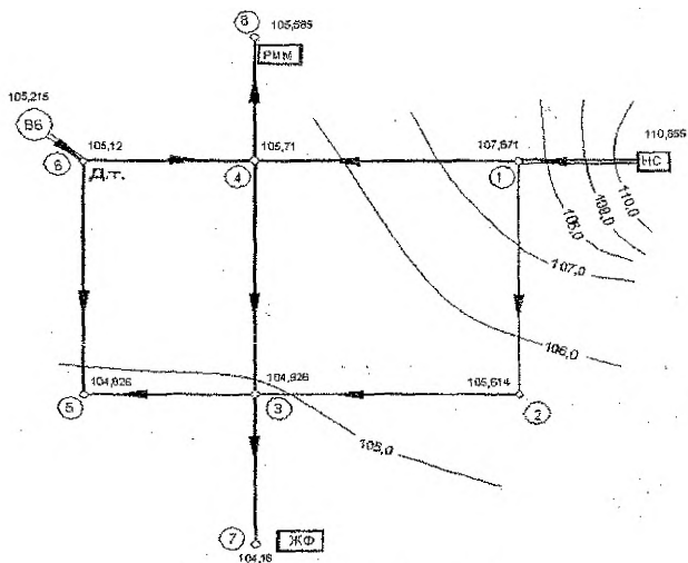
Рис. 3.3 – Карта пьезолиний
