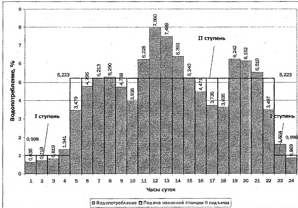
Рис. 1.1 – Сводный график водопотребления, совмещенный с графиком подачи насосной станции II подъема
