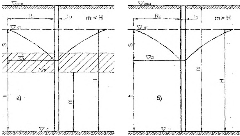
Рис. 6.1 – Водозаборные скважины: а) в напорном пласте; б) в безнапорном пласте
