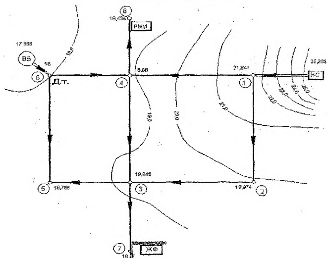
Рис. 3.4 – Карта свободных напоров
