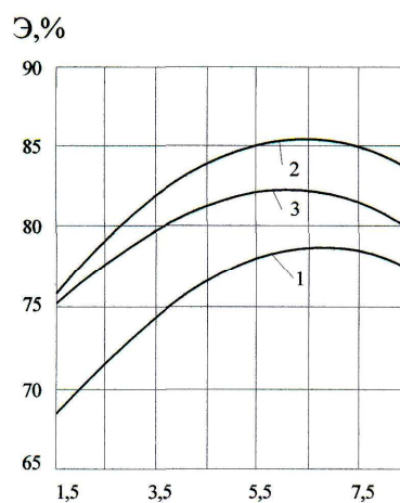
Рис. 2. Влияние дозы алюминия на эффект комплексного электрохимического обесцвечивания воды. 1, 2, 3 – плотность тока на нерастворимых электродах соответственно 15, 20, 25 mA/cm^2
